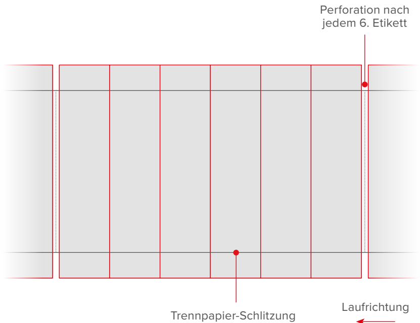
Trennpapierschlitzung, Partitionen möglich
