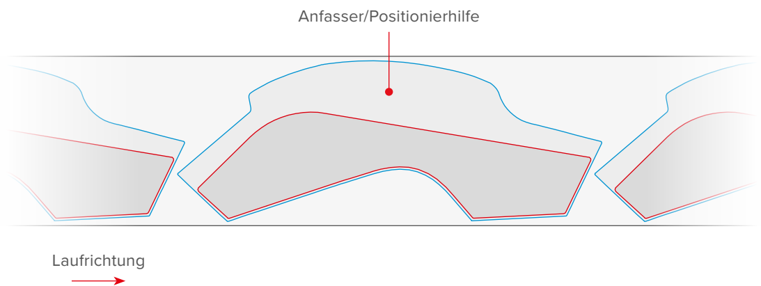
Stanzteile materialsparend verschachtelt
